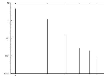
(a) Eigenvalues
